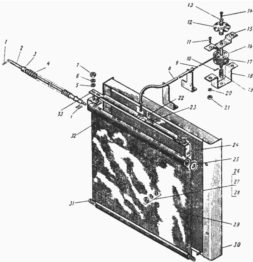
Рис. 28. Шторка
