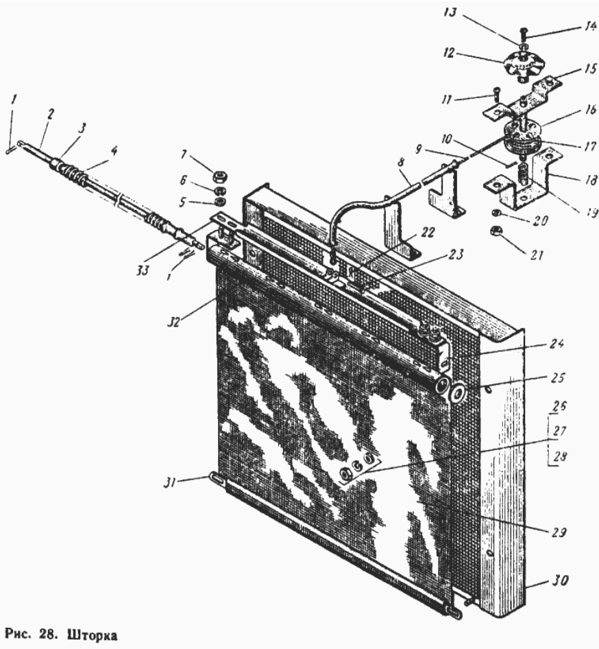
ЮМЗ-6Л Рис. 28. Шторка.
