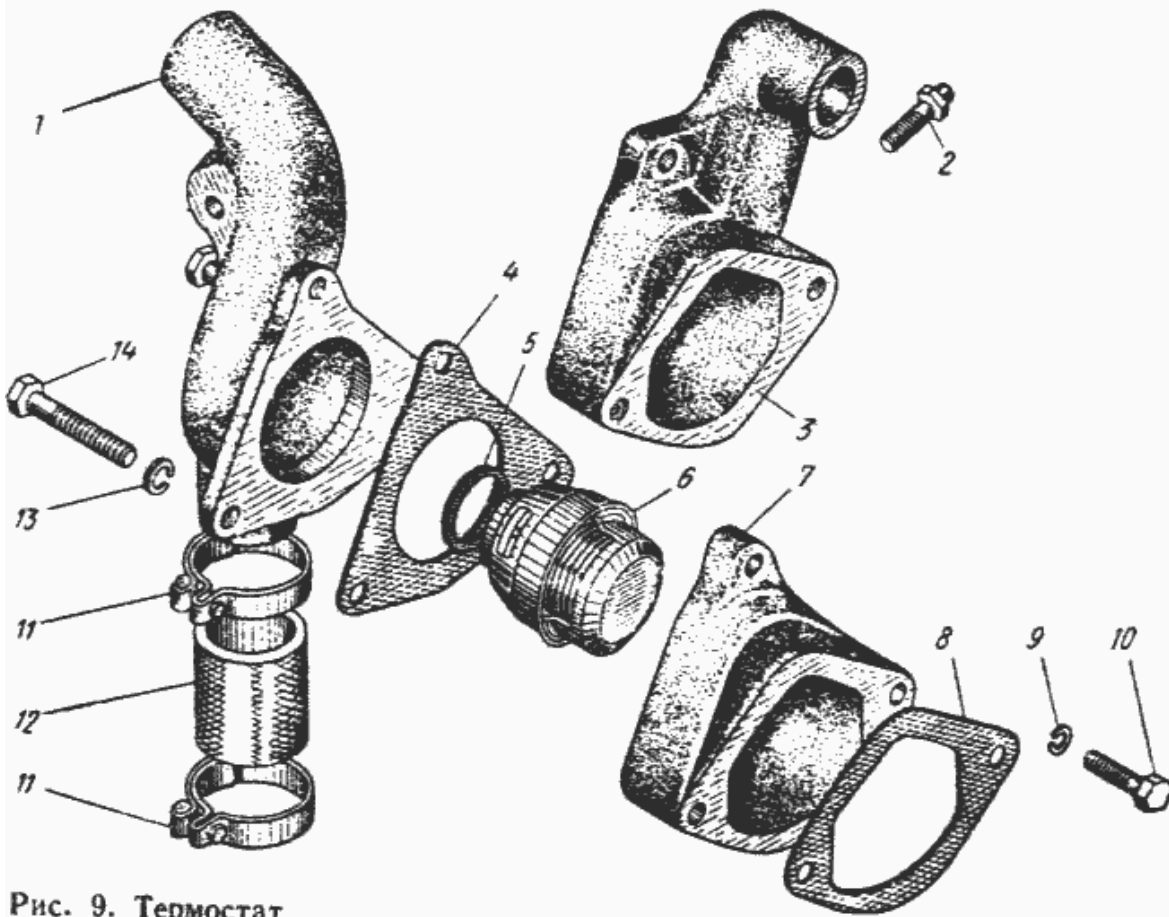
ЮМЗ-6Л Рис. 09. Термостат.
