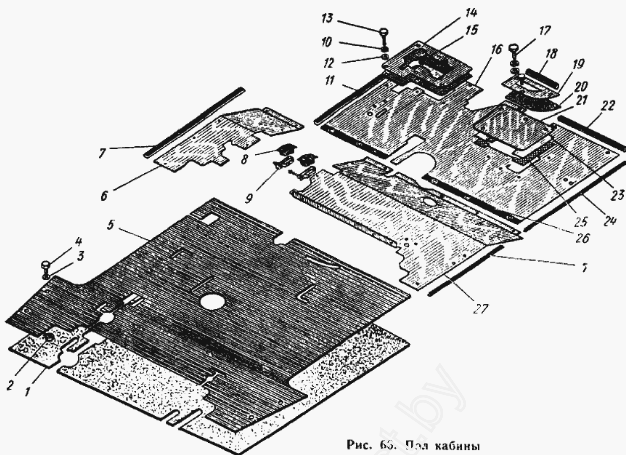
ЮМЗ-6Л Рис. 66. Пол кабины.
