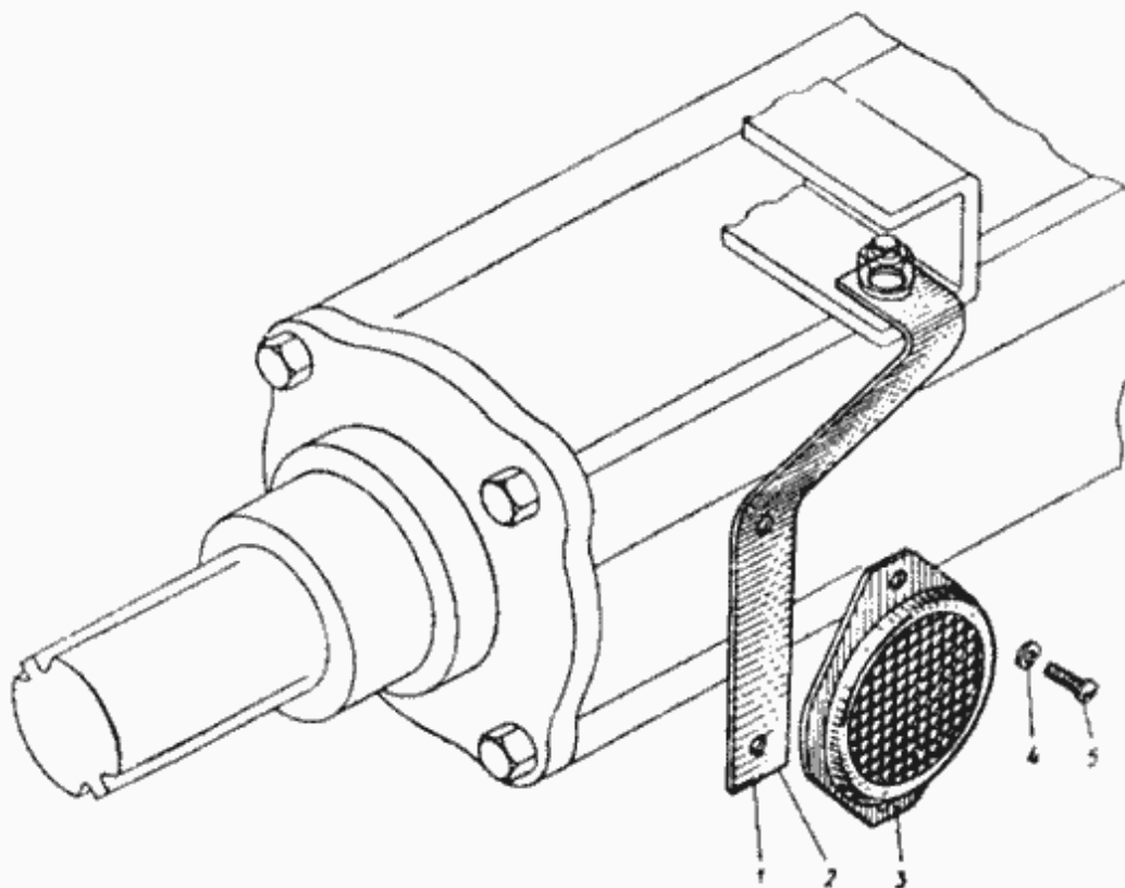
Рис. 52. Отражатели
