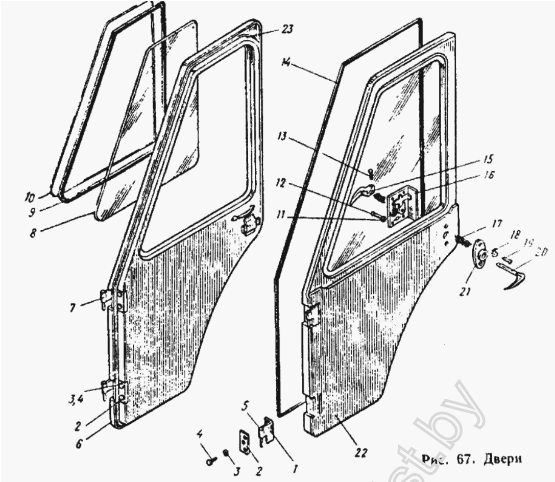
ЮМЗ-6Л Рис. 67. Двери.
