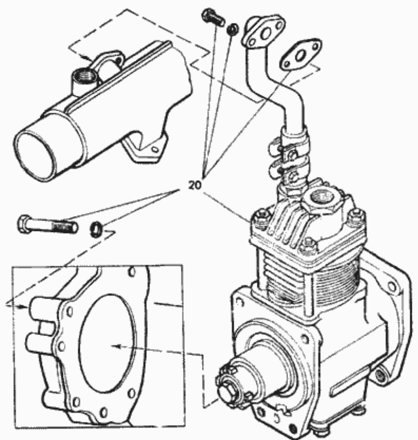
Рис. 15. Дизели Д144-0000100-34, Д144-0000100-38
