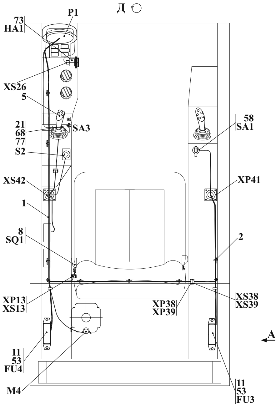
Рис. 24 211.50.18.000 Электрическая система кабины Fig. 24 Electric system of the cab Fig. 24 Système électrique de la cabine Fig. 24 Sistema eléctrico de la cabina
