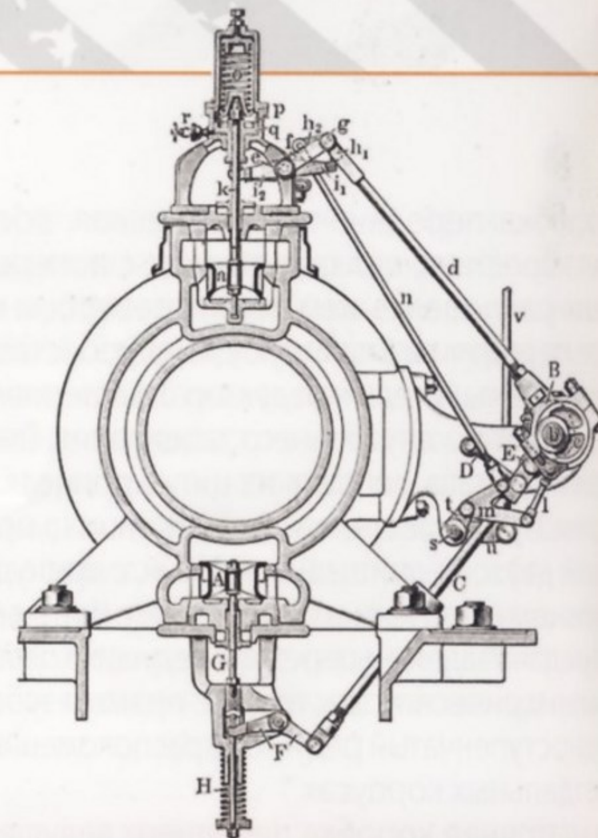
Двигатель фирмы Sulzer.
